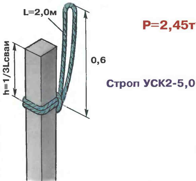
3. Железобетонная свая
