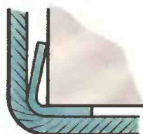
Загнутые прокладки из листового материала
