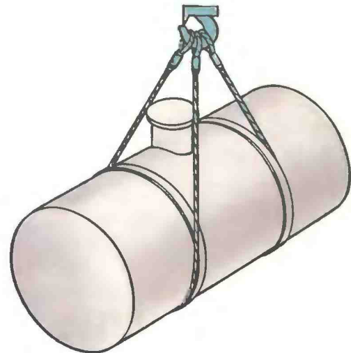
СТРОПОВКА ЦИЛИНДРИЧЕСКОГО РЕЗЕРВАРА ДВУМЯ ДВУХПЕТЛЕВЫМИ СТРОПАМИ
