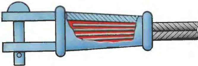
Заливкой
