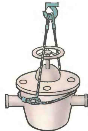
СТРОПОВКА ЗАДВИЖКИ ДВУХПЕТЛЕВЫМ СТРОПОМ
