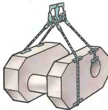
СТРОПОВКА ДЕТАЛИ СТАНКА ДВУМЯ ДВУХПЕТЛЕВЫМИ СТРОПАМИ
